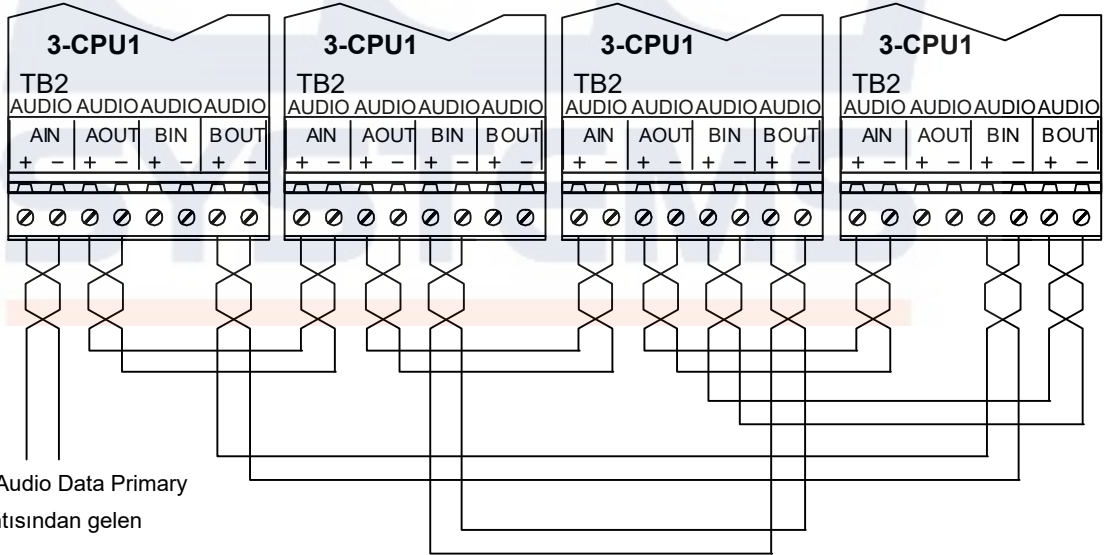
Class A network riser hat bağlantı şeması
