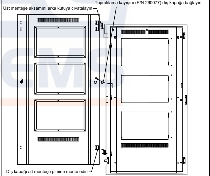
EST3 DIŞ KAPAK MONTAJ DETAYI
