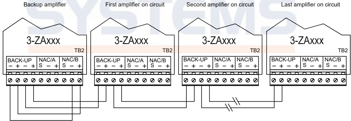
Sembolik yedek amplifikatör kablolama
