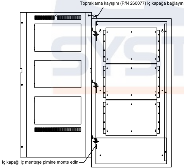
EST3 İÇ KAPAK MONTAJ DETAYI
