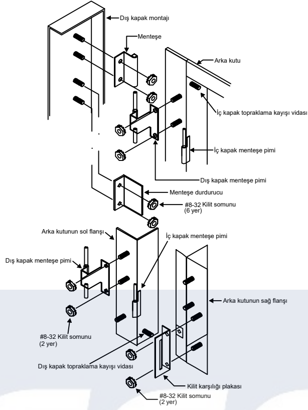
EST3 VİDALAMA DETAYLARI
